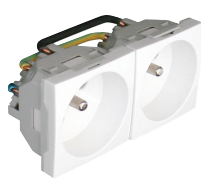
97. 2 x gniazdo z uziemieniem z zabezpieczeniem przed dziećmi pod kątem 45°
