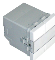
34. Czterokrotny przycisk sensorowy niskonapięciowy 12V - 50mA / 32V - 18mA
